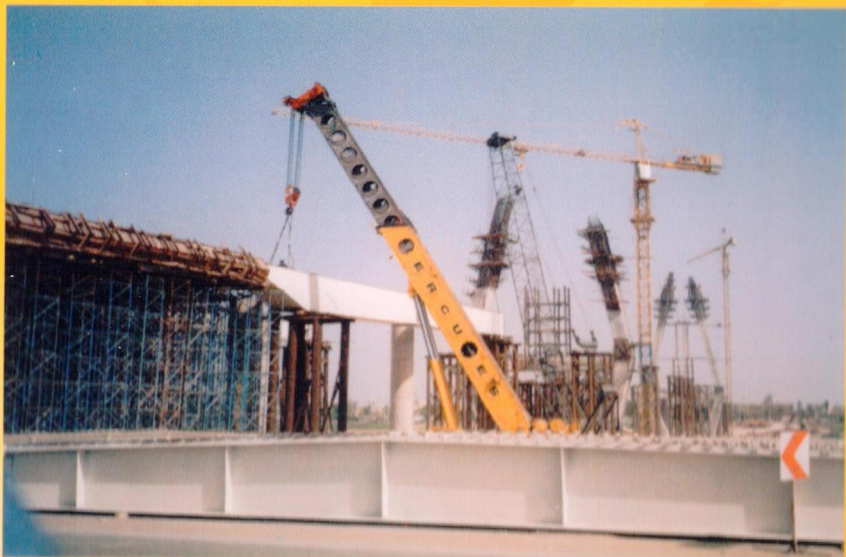
• نصب تیرهای اصلی پل هشتم اهواز
